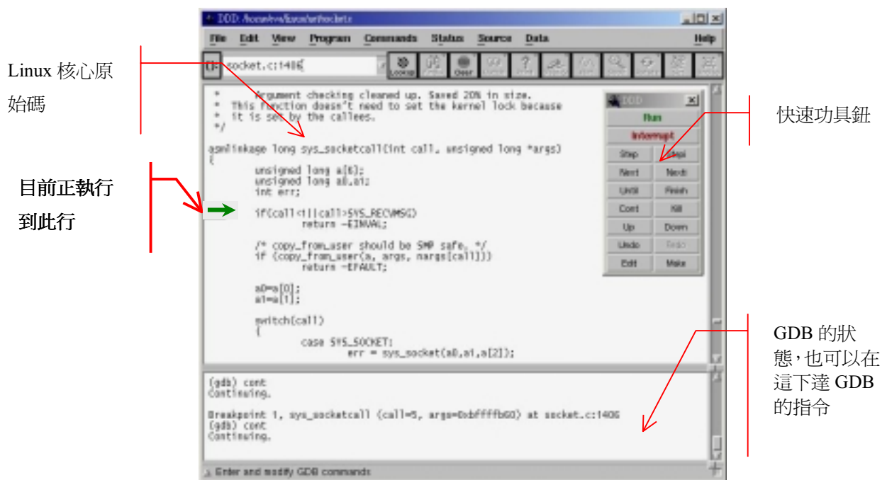
圖四：DDD 除錯畫面
