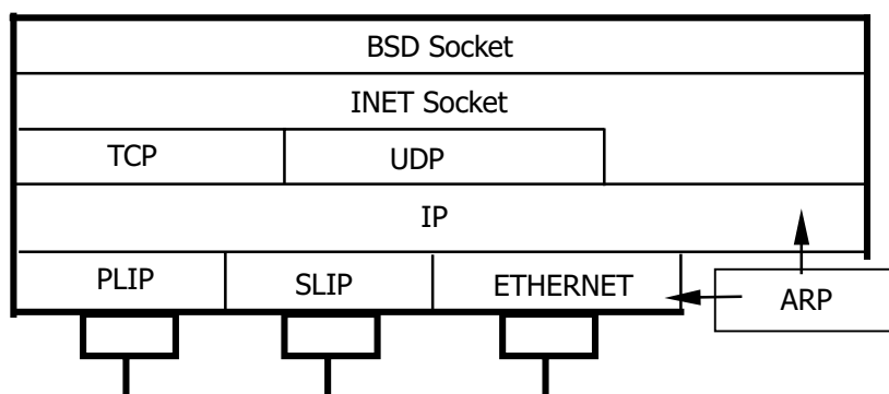
圖一：網路分層架構
