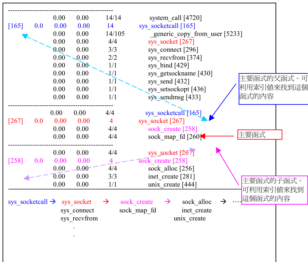
圖五：KernProf 報告檔
