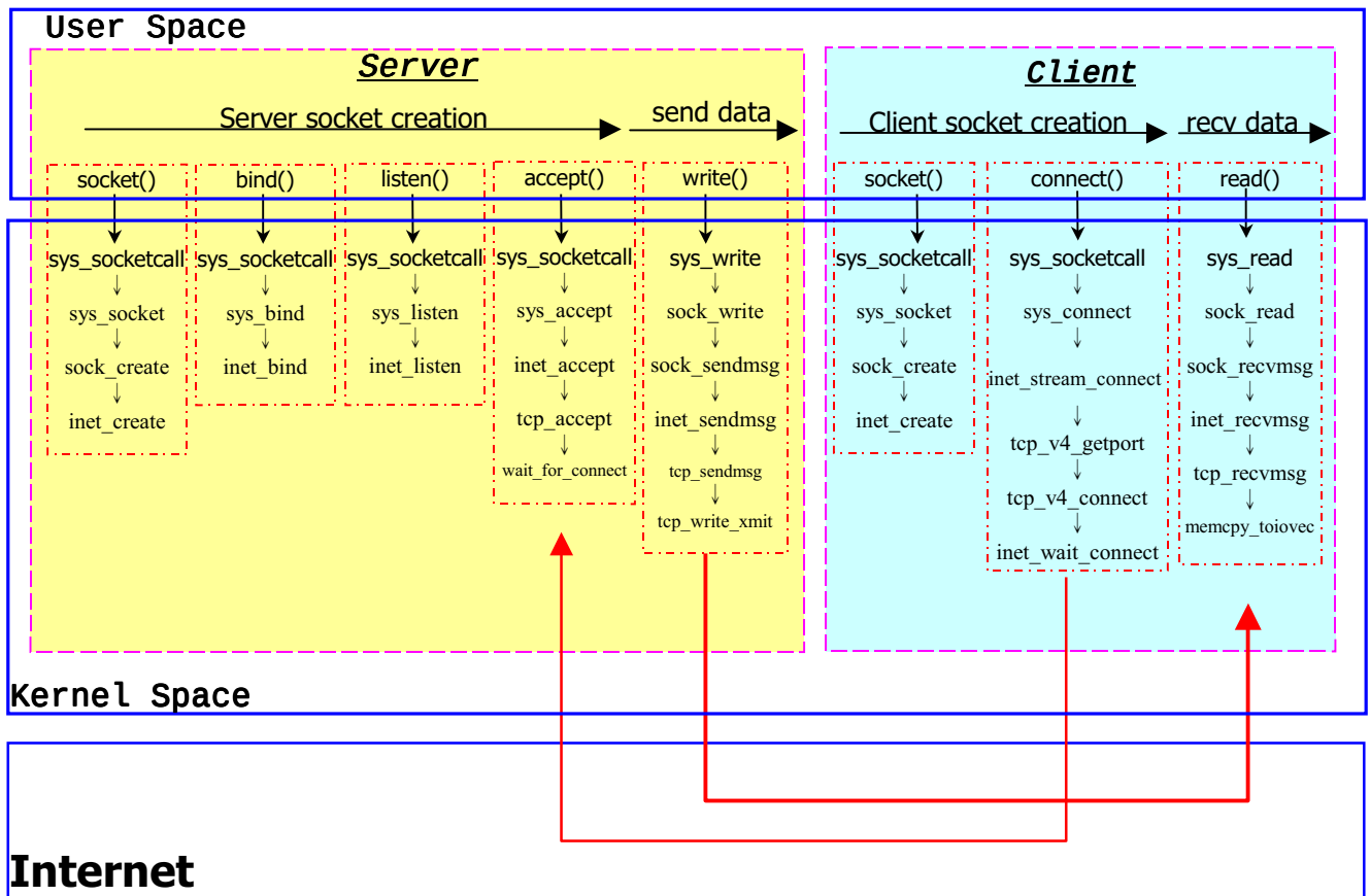
圖六：由 Server 送資料到 Client 的過程
