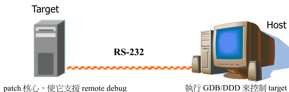
圖二：遠端除錯示意圖
