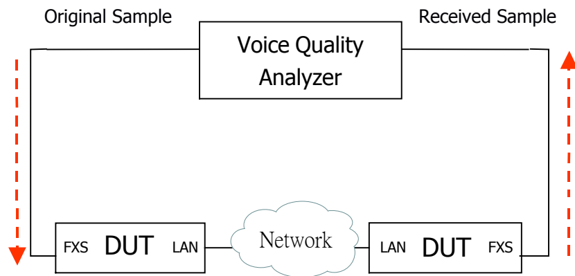
圖 3-1. Gateway 語音品質測試組態
