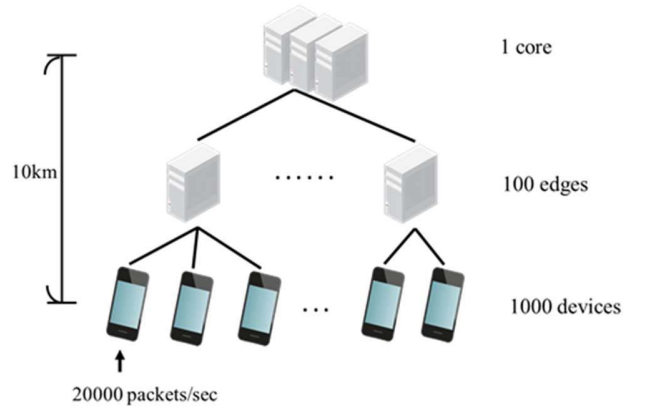
Fig. 6. Simulation scenario.
